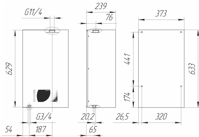
Рисунок 4. Габаритные и присоединительные размеры
