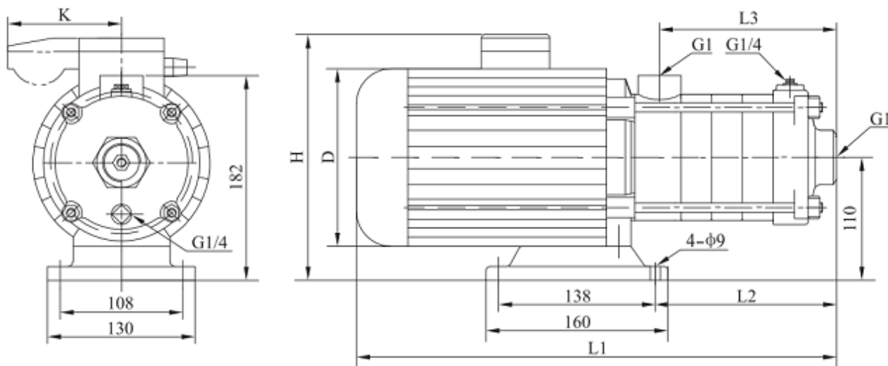
Габаритно-присоединительные размеры
